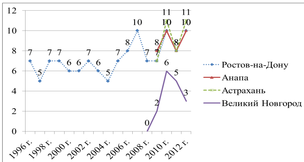
Рис. 1. Число возможных генераций дирофилярий в комарах
